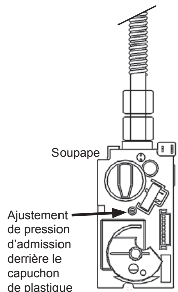
Assemblage de la soupape
