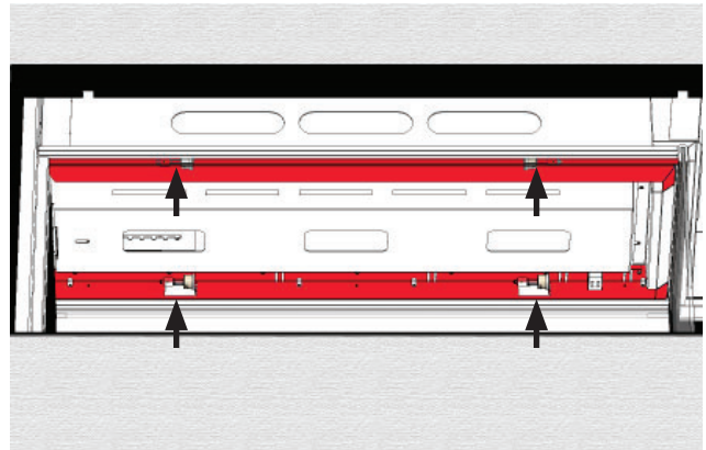
LX1 Péninsule : deux rails de 2 lampes chacun Emplacement des lampes en regardant vers le haut dans la boîte de foyer
