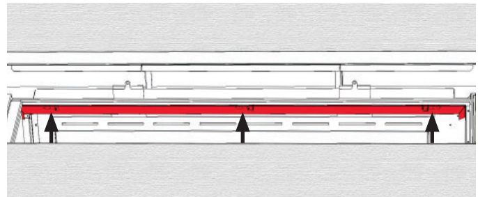
LX2 à 3 faces et LX2 d'angle : un rail de 3 lampes Emplacement des lampes en regardant vers le haut dans la boîte de foyer
