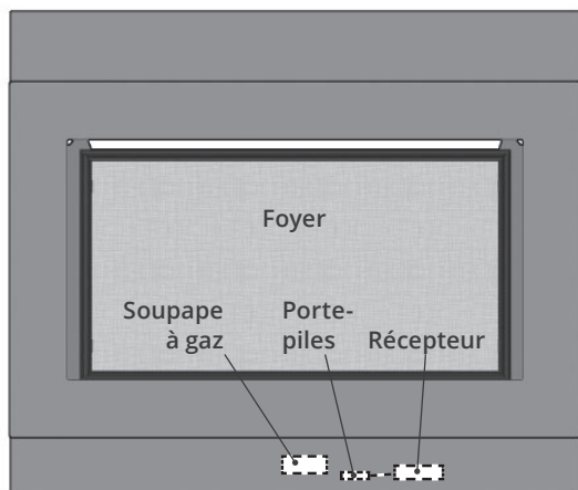
Porte-piles situé à côté du récepteur sous la boîte de foyer derrière la bordure.
