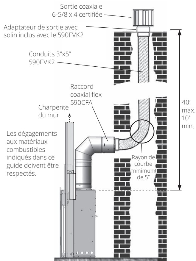
Installation coaxiale flex 3x5 à la cheminée incombustible existante—Conversion à la cheminée
