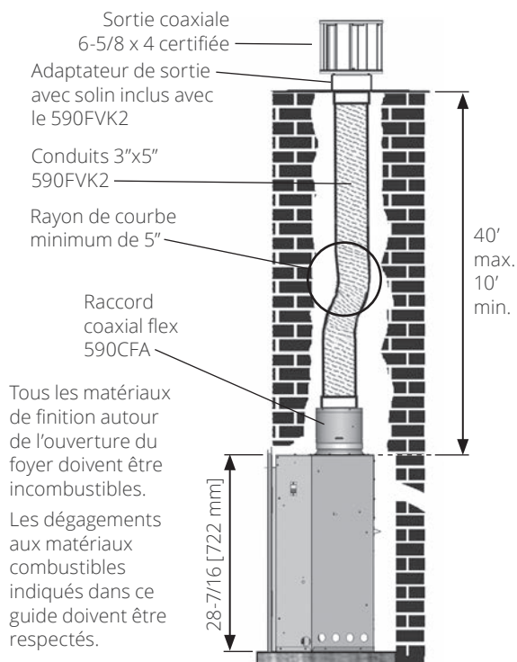
Installation coaxiale flex 3x5 entièrement dans le foyer incombustible existant—conversion à l'appareil
