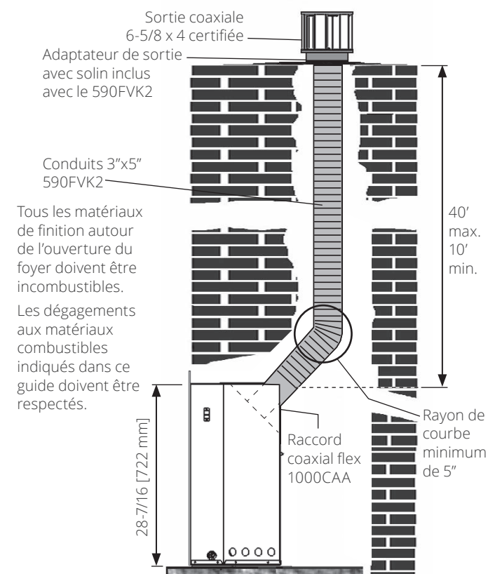
Installation coaxiale flex 3 x 5 entièrement dans le foyer incombustible existant - conversion à l'appareil
