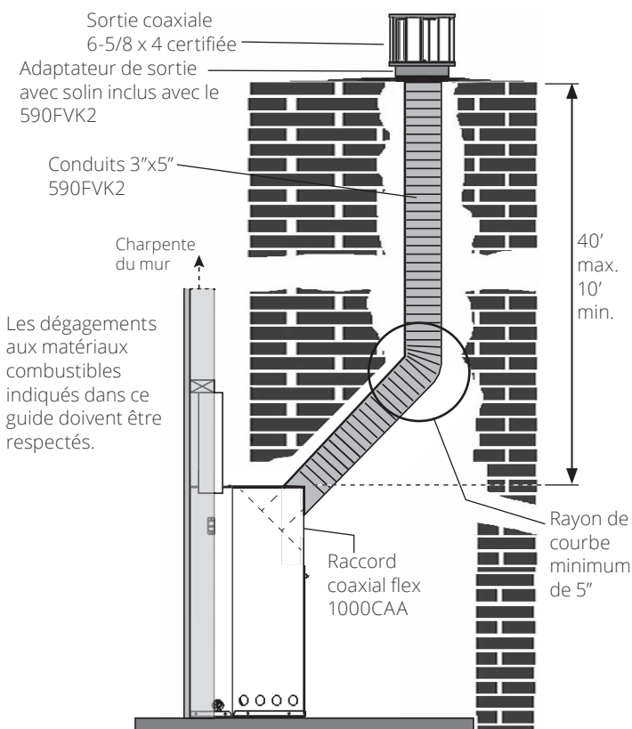
Installation coaxiale flex 3x5 partiellement dans le foyer incombustible existant - conversion à l'appareil
