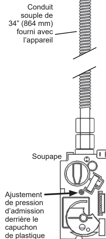
Assemblage de la soupape
