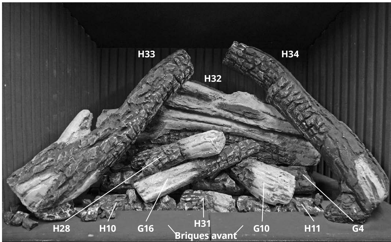
Bûches traditionnelles 1000LSKV2 installées
