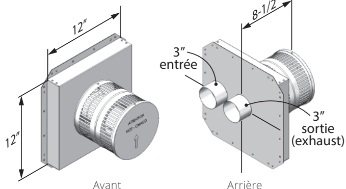
Sortie murale colinéaire
